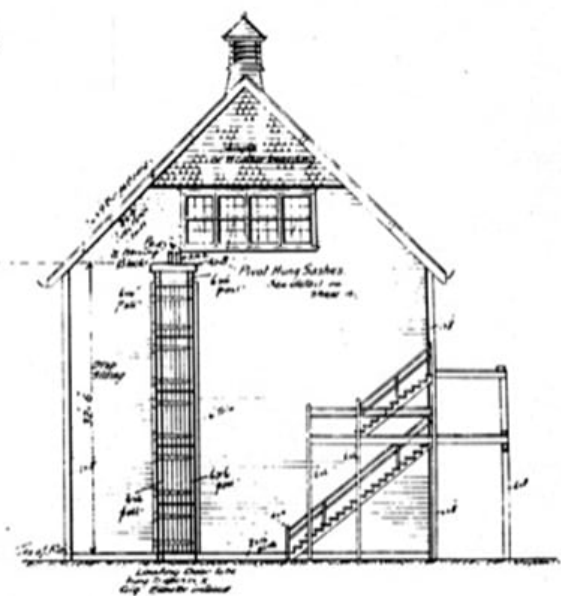
END ELEVATION
